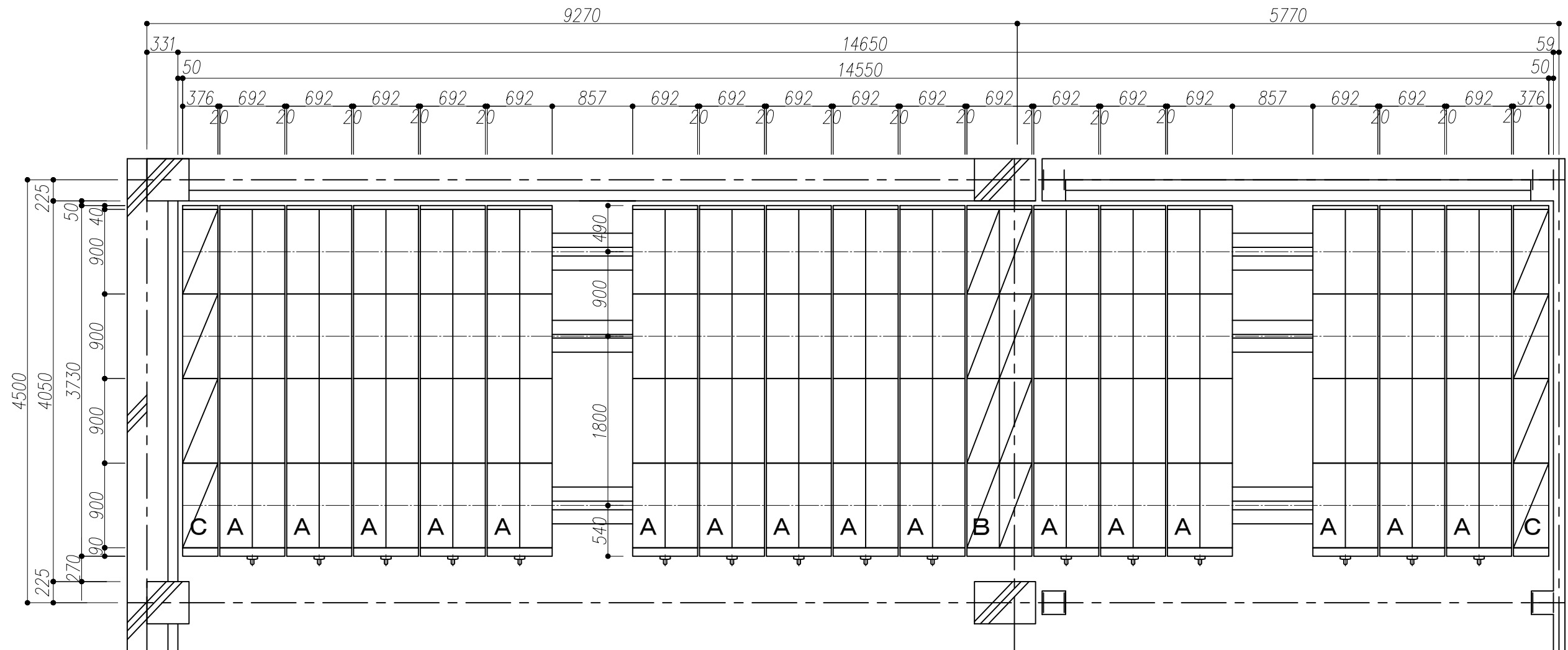
1階 書庫 制震ハンドル式スタックランナー 配置図 S=1/50
