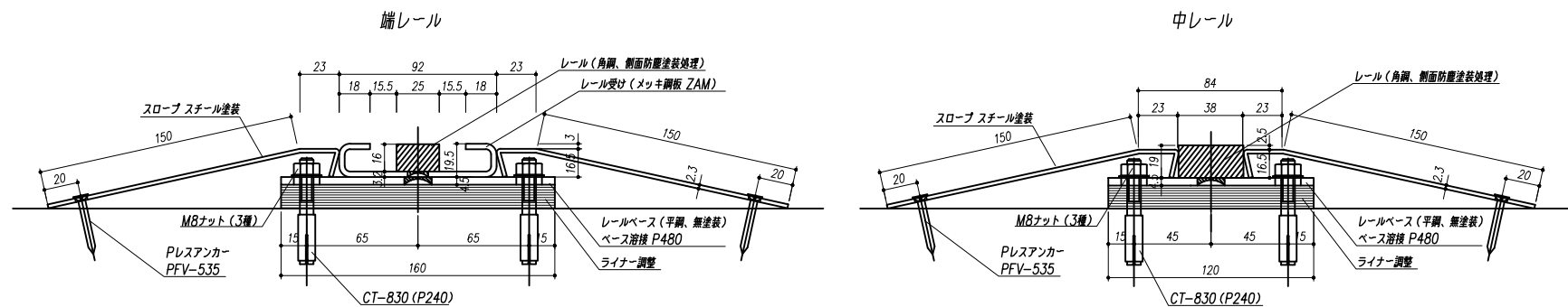
露出式レール 断面詳細図 S=1/4
