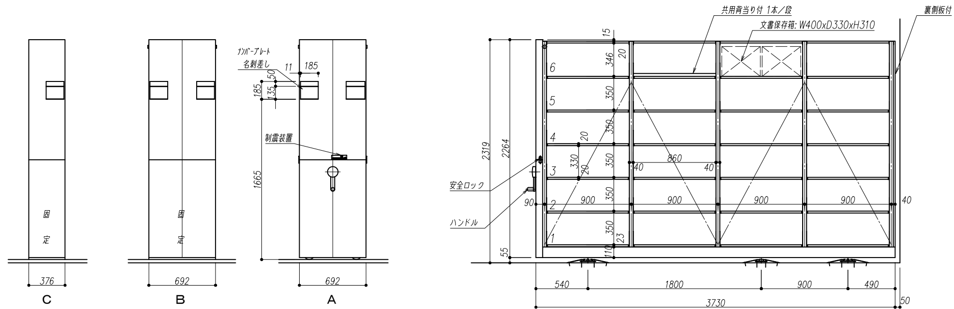
1階 書庫 制震ハンドル式スタックランナー 姿図 S=1/40
